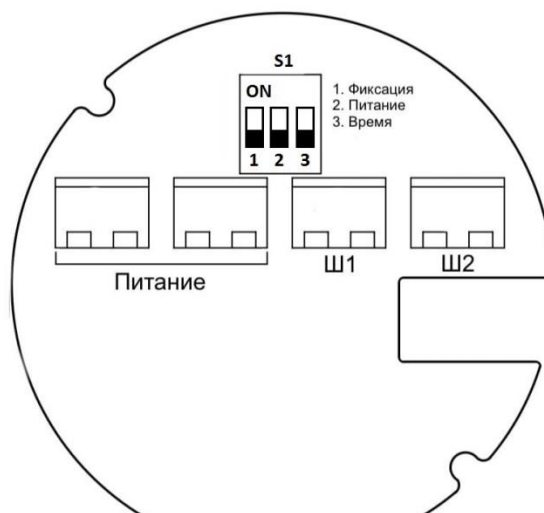
Рисунок 2 – Расположение элементов коммутации и управления на плате
